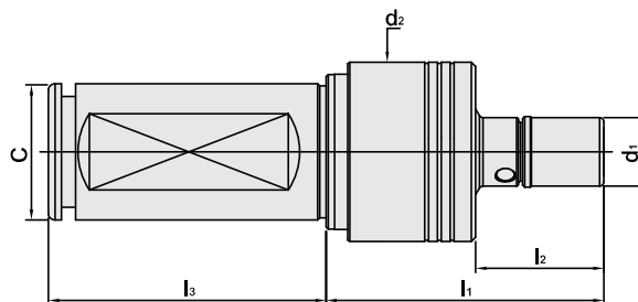
直柄 STA 同步補償攻牙刀桿
