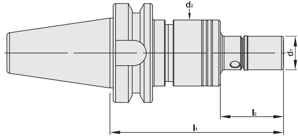
BT / STA 同步補償攻牙刀桿
