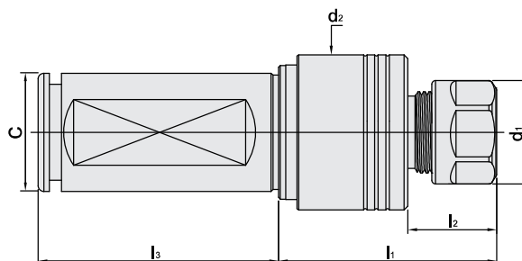
直柄 STA 同步補償攻牙刀桿
