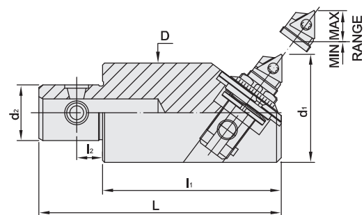
SCK / BYB 微切削搪刀柄
